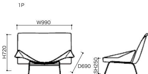
●正面図 (単位:mm)
